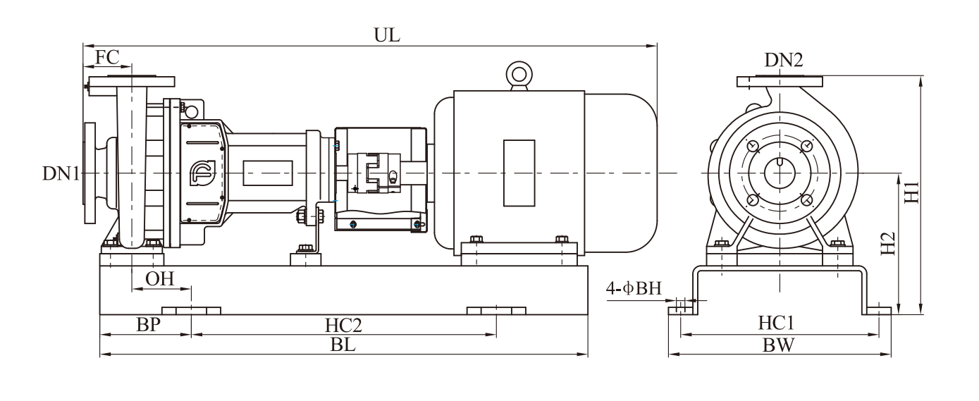
Габаритно-присоединительные размеры насосного агрегата в сборе NISO
