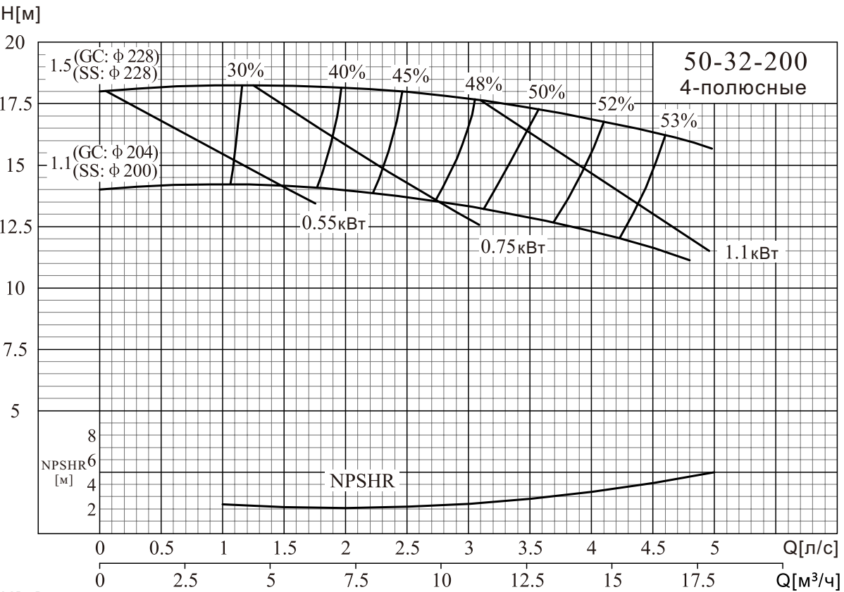
NISO,NIS,NISF 50-32-200/65-40-200
