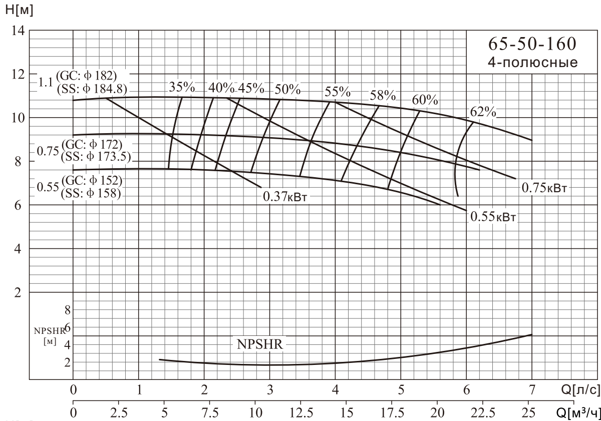
NISO,NIS,NISF 65-50-160/80-50-200
