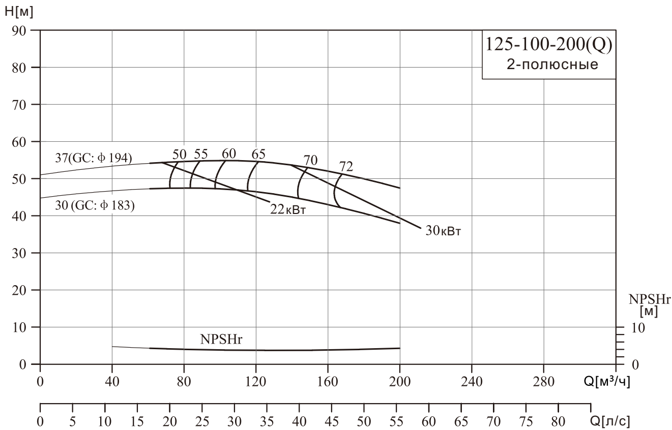
NIS125-100-200(Q)/125-100-200G
