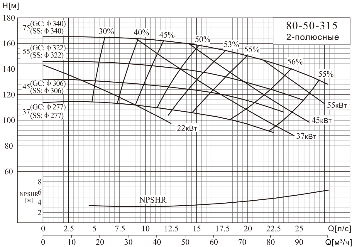
NISO,NIS,NISF 80-50-315/80-65-160
