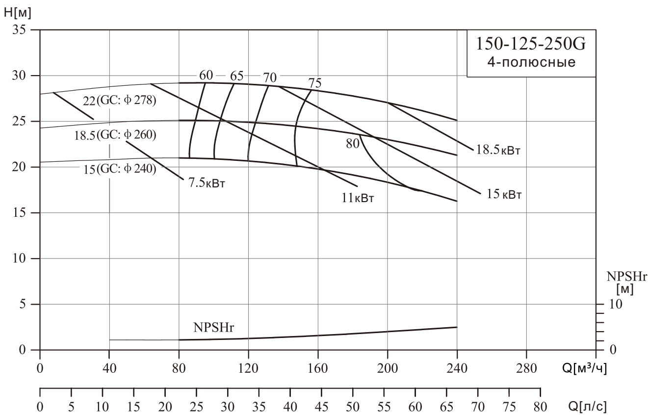
NIS150-125-250G/150-125-315(Q)
