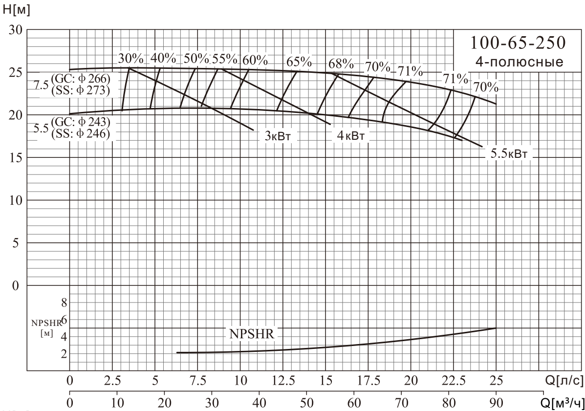
NISO,NIS,NISF 100-65-250/100-65-315
