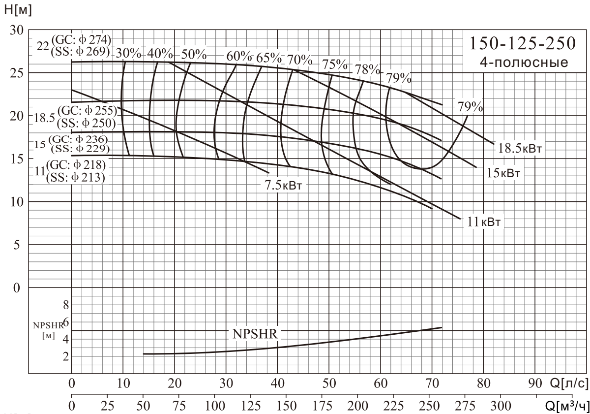
NISO,NIS,NISF 150-125-250/150-125-315
