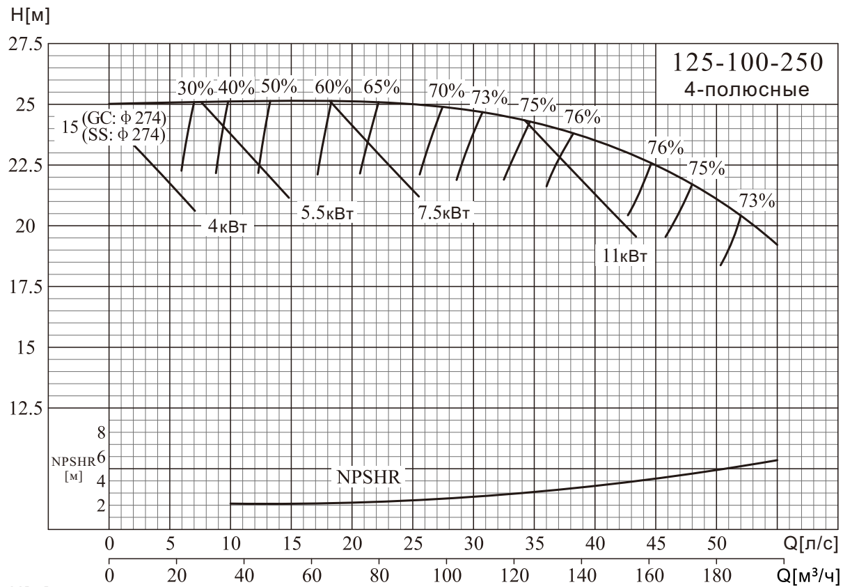
NISO,NIS,NISF 125-100-250/125-100-315
