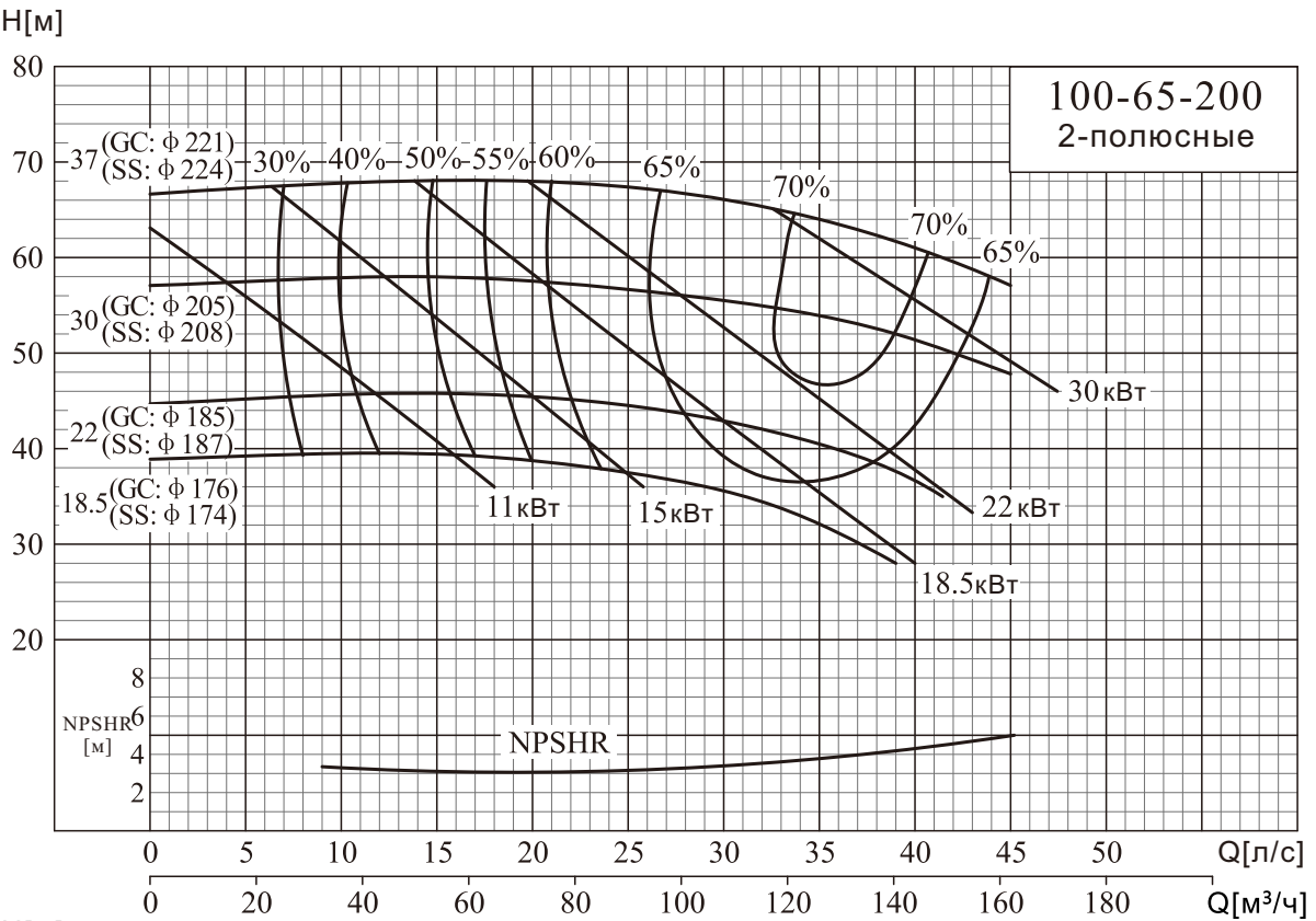
NISO,NIS,NISF 100-65-200/100-65-250
