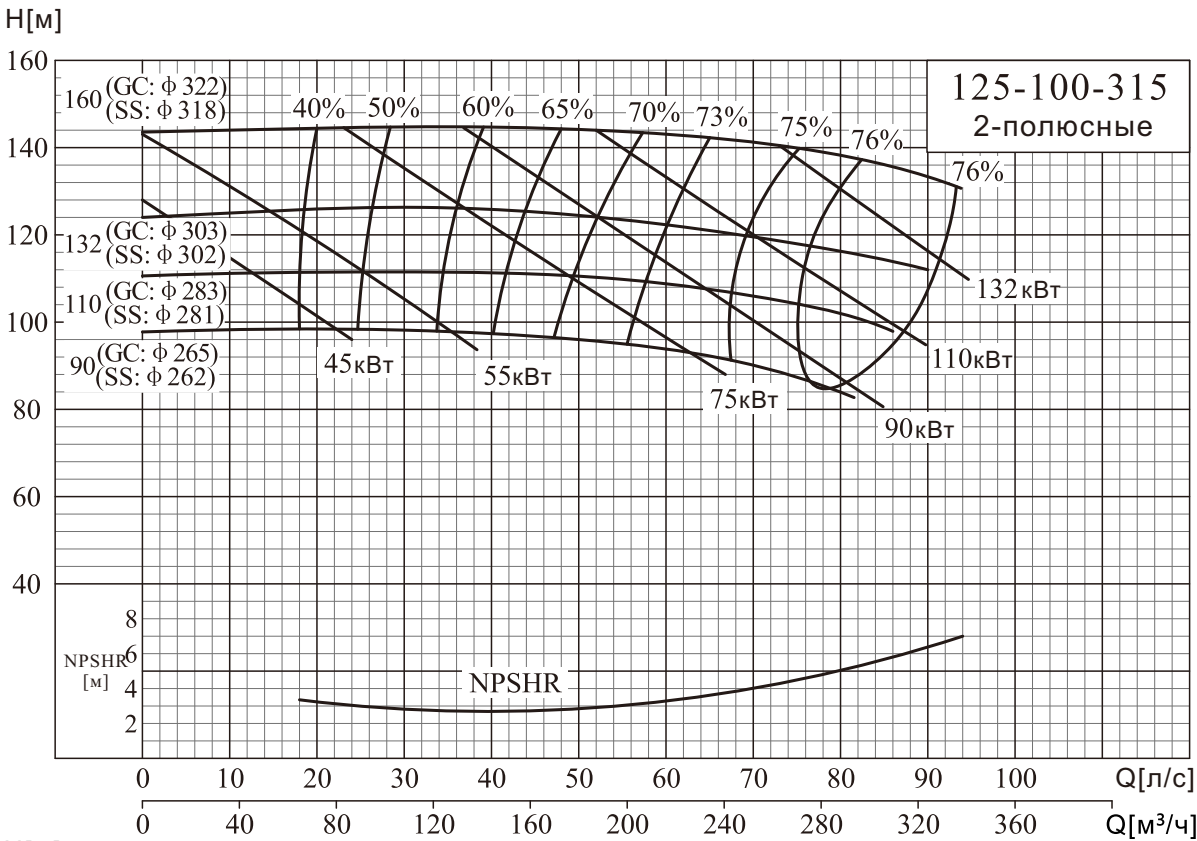
NISO,NIS,NISF 125-100-315/50-32-160
