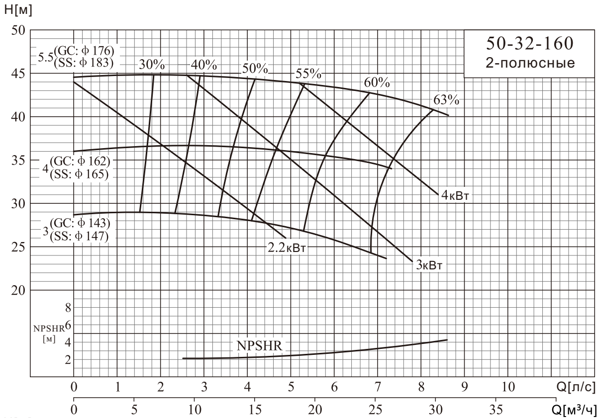
NISO,NIS,NISF 50-32-160/50-32-200
