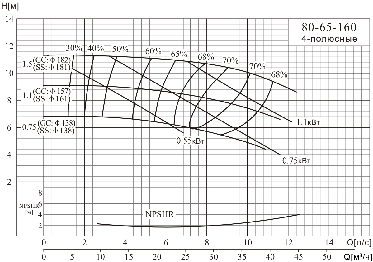
NISO,NIS,NISF 80-65-160/100-65-200
