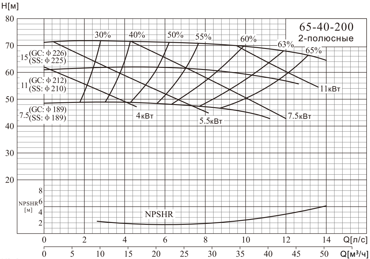
NISO,NIS,NISF 65-40-200/65-40-250
