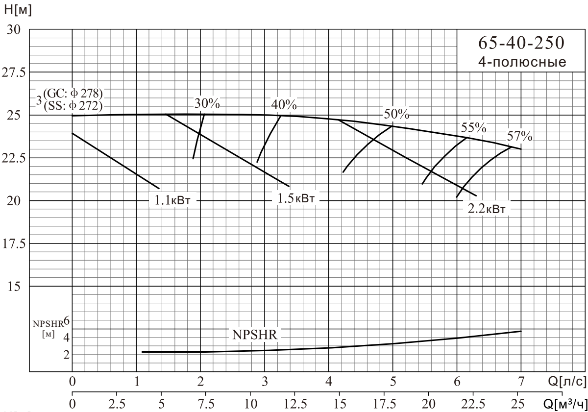
NISO,NIS,NISF 65-40-250/65-40-315
