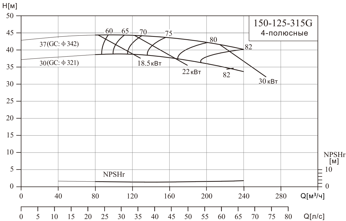
NIS150-125-315G/150-125-400(Q)
