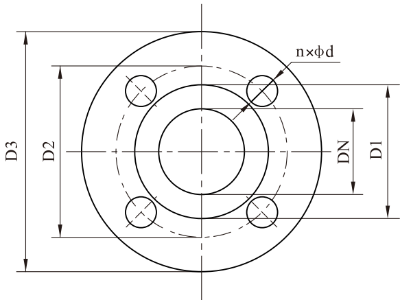
Размеры фланцев NIS*G,NIS*(Q)
