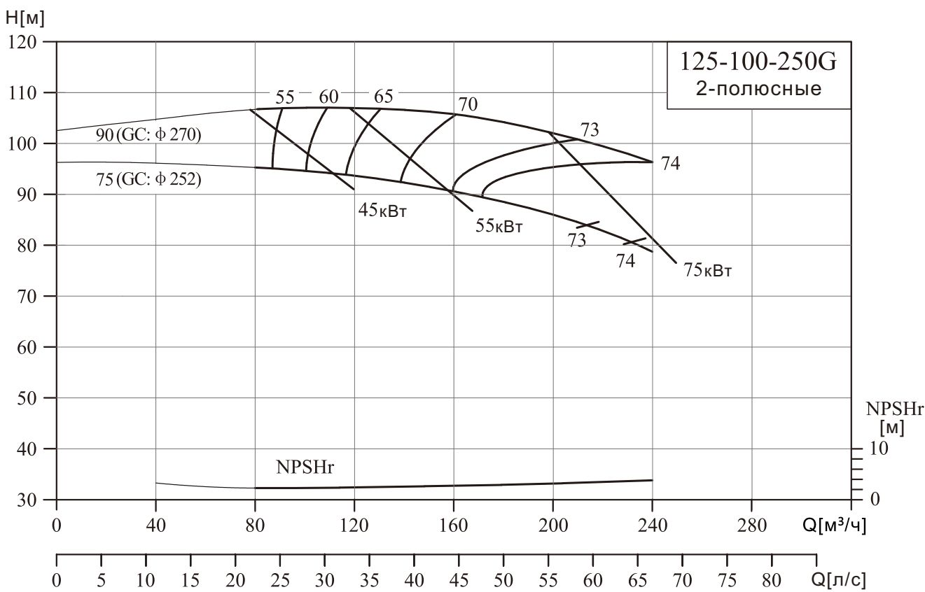
NIS125-100-250G/125-100-315G
