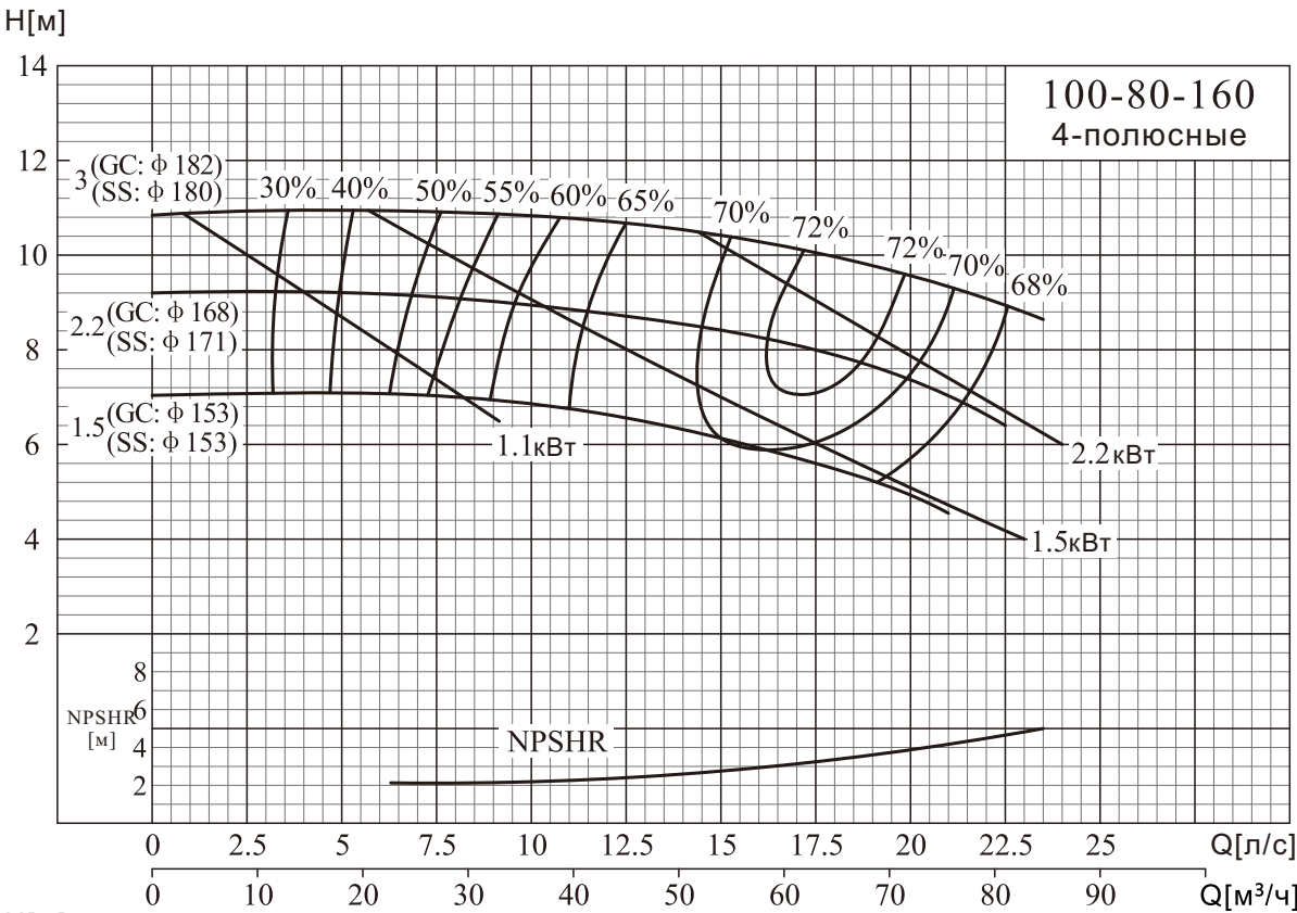
NISO,NIS,NISF 100-80-160/125-100-200
