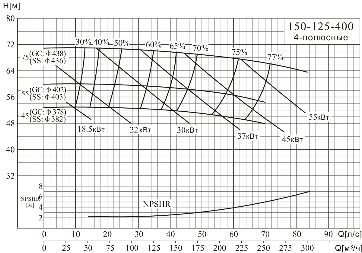
NISO,NIS,NISF 150-125-400/200-150-315
