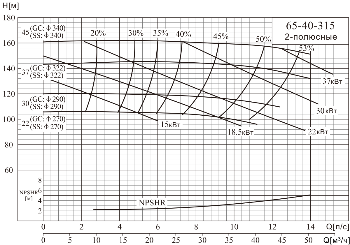
NISO,NIS,NISF 65-40-315/65-50-160
