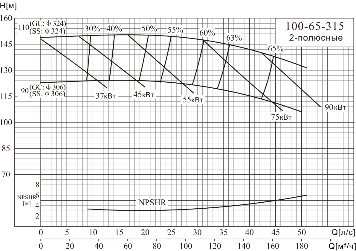
NISO,NIS,NISF100-65-315/100-80-160
