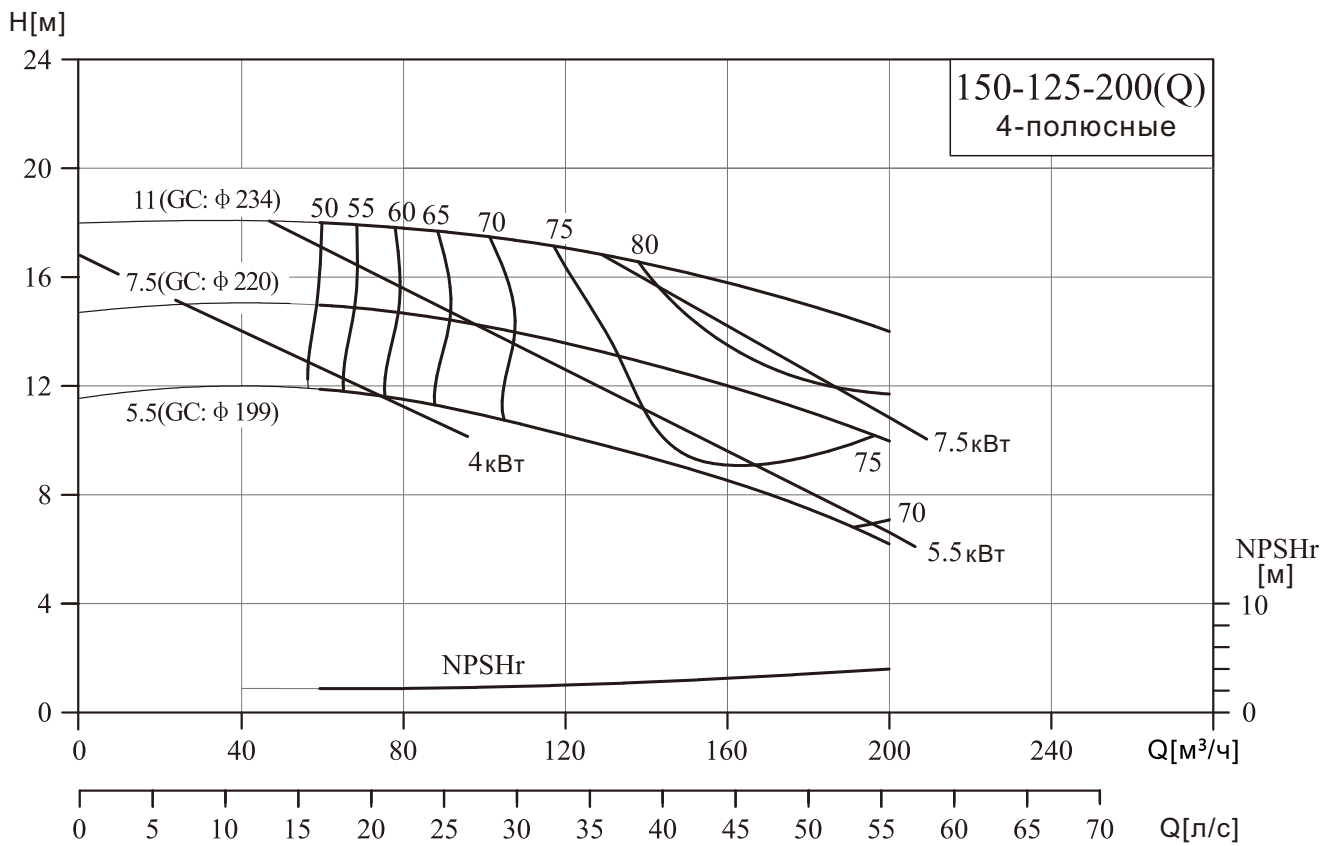
NIS150-125-200(Q)/150-125-200G
