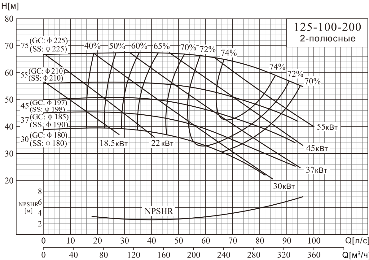
NISO,NIS,NISF125-100-200/125-100-250
