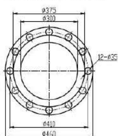
Фланец ВХОДА ВОДЫ GB/T17241.7-1998 PN 1.6MPa
