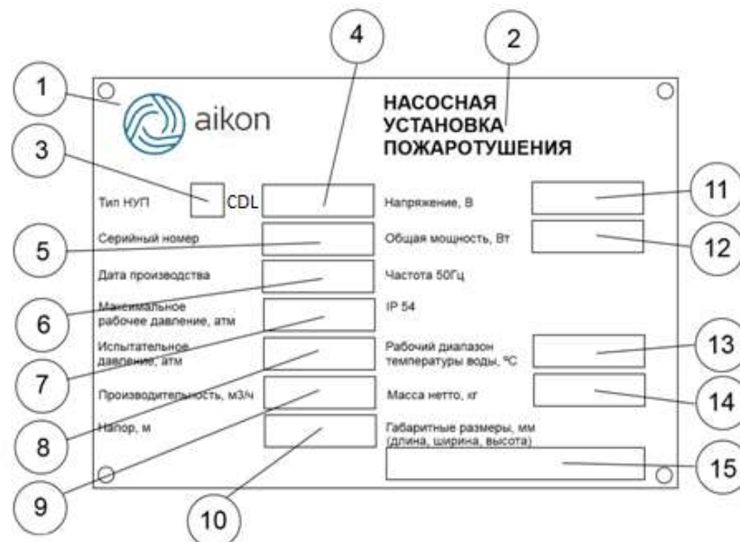
Рис. 2 Маркировочная табличка
